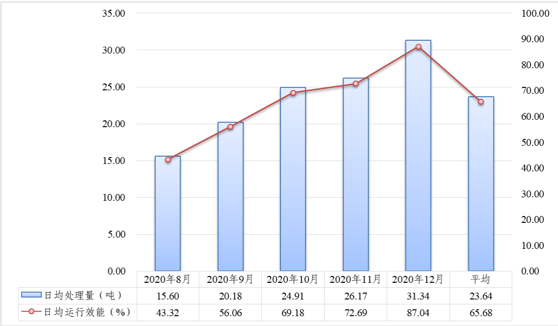
图 1 德兴厨余生物质处理站日均处理量和运行效能分析
