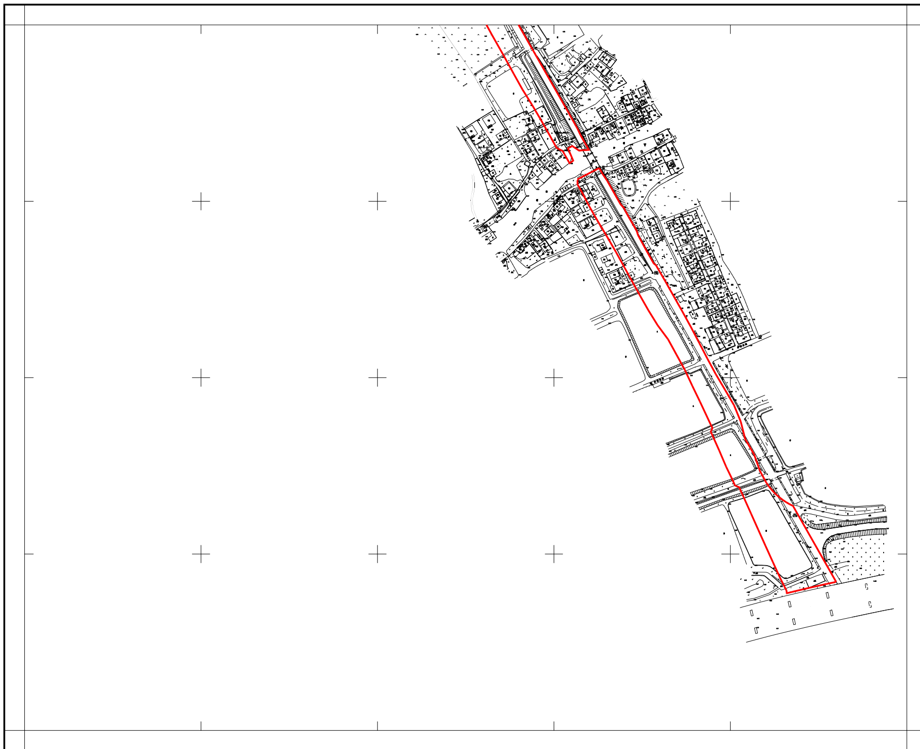
S296(海鸥公路) 扩建工程拟征地红线图-5
