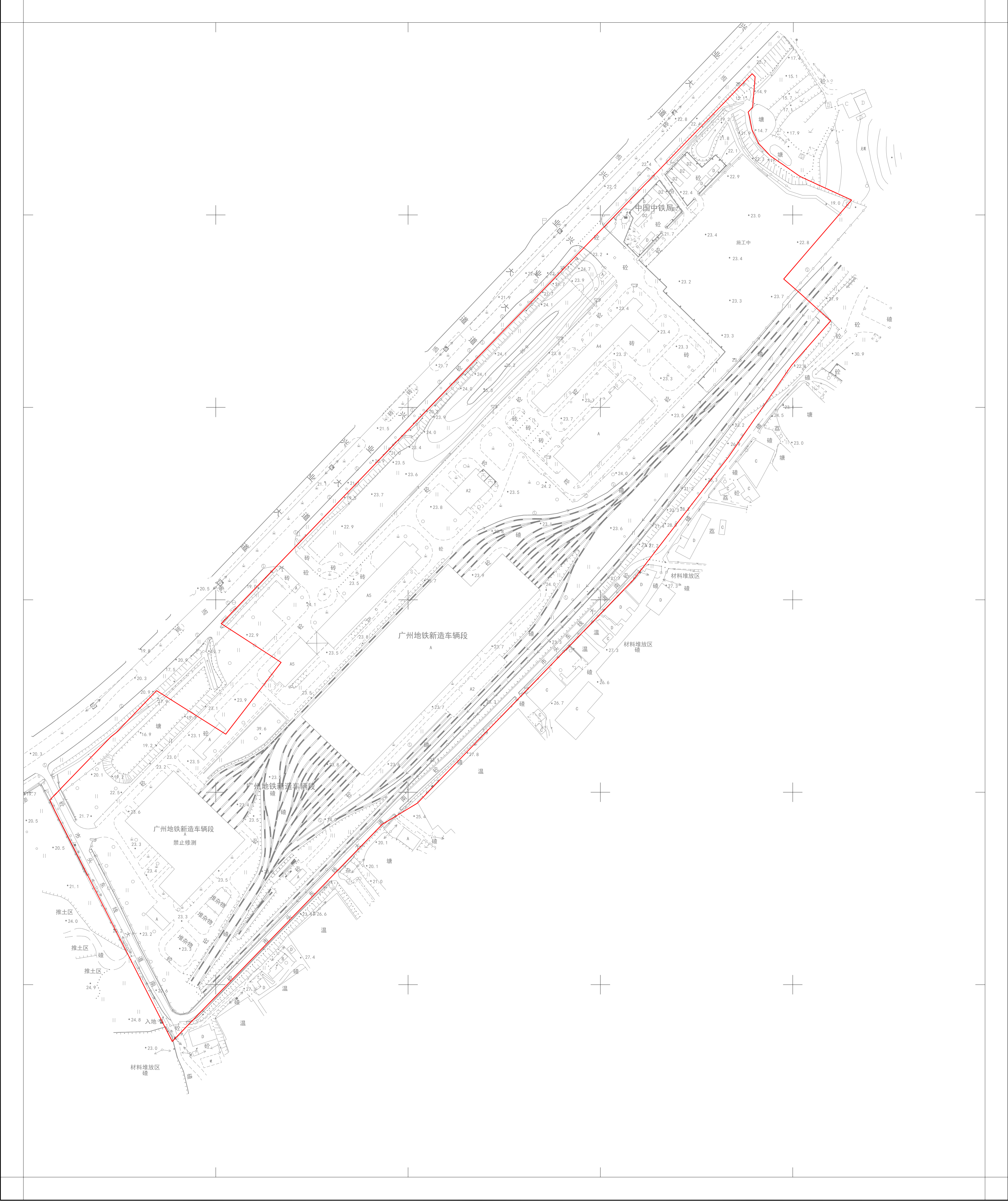
广州市轨道交通四号线新造车辆段拟征地红线图
