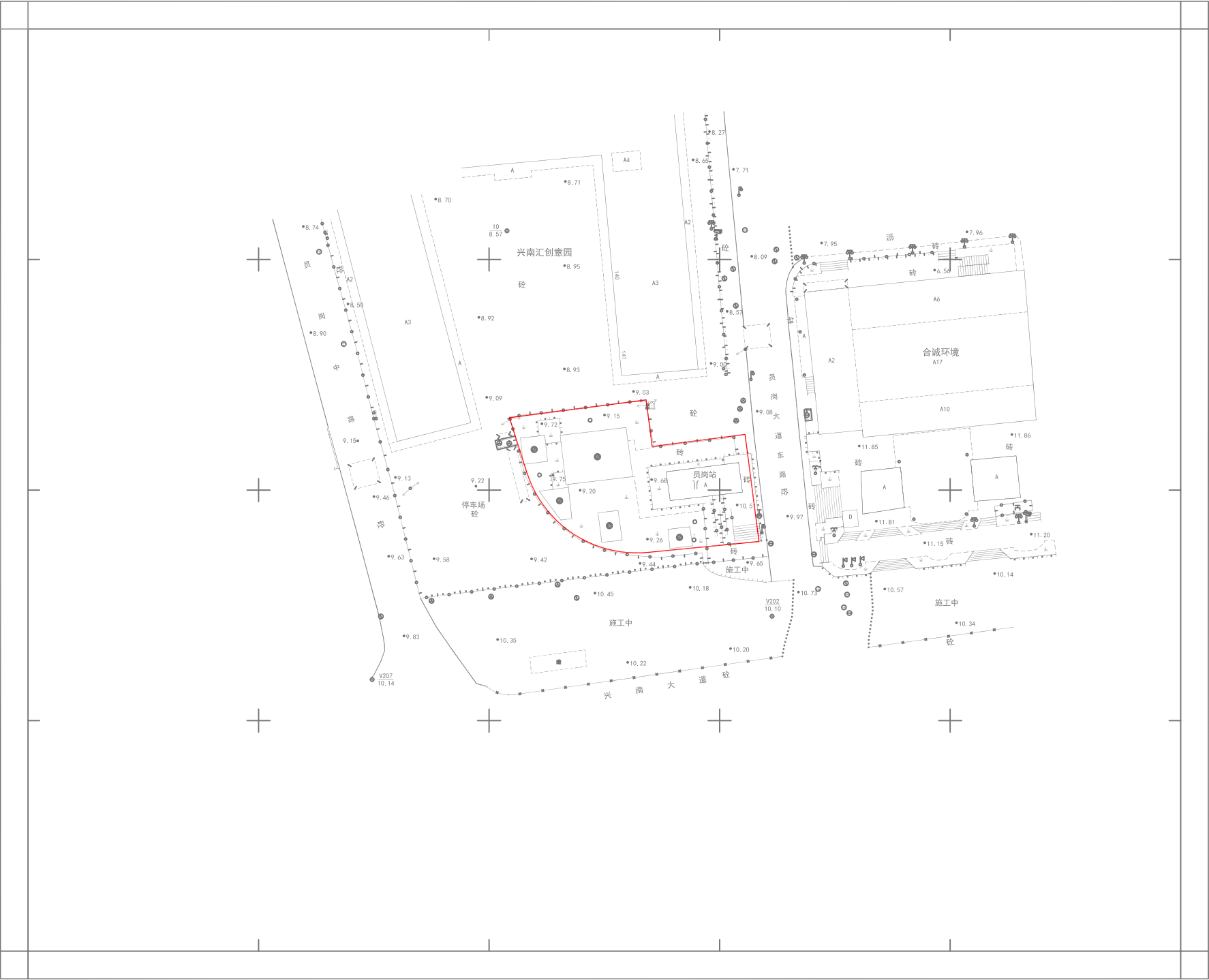
广州市番禺区2024年度第五十八批次城镇建设用 〔广州市轨道交通七号线一期钟村站附属工程、万博站-官堂站区间风井、员岗站(原官堂站)地面附属设施、板桥站附属工程项目地块一〕拟征地红线图(三)
