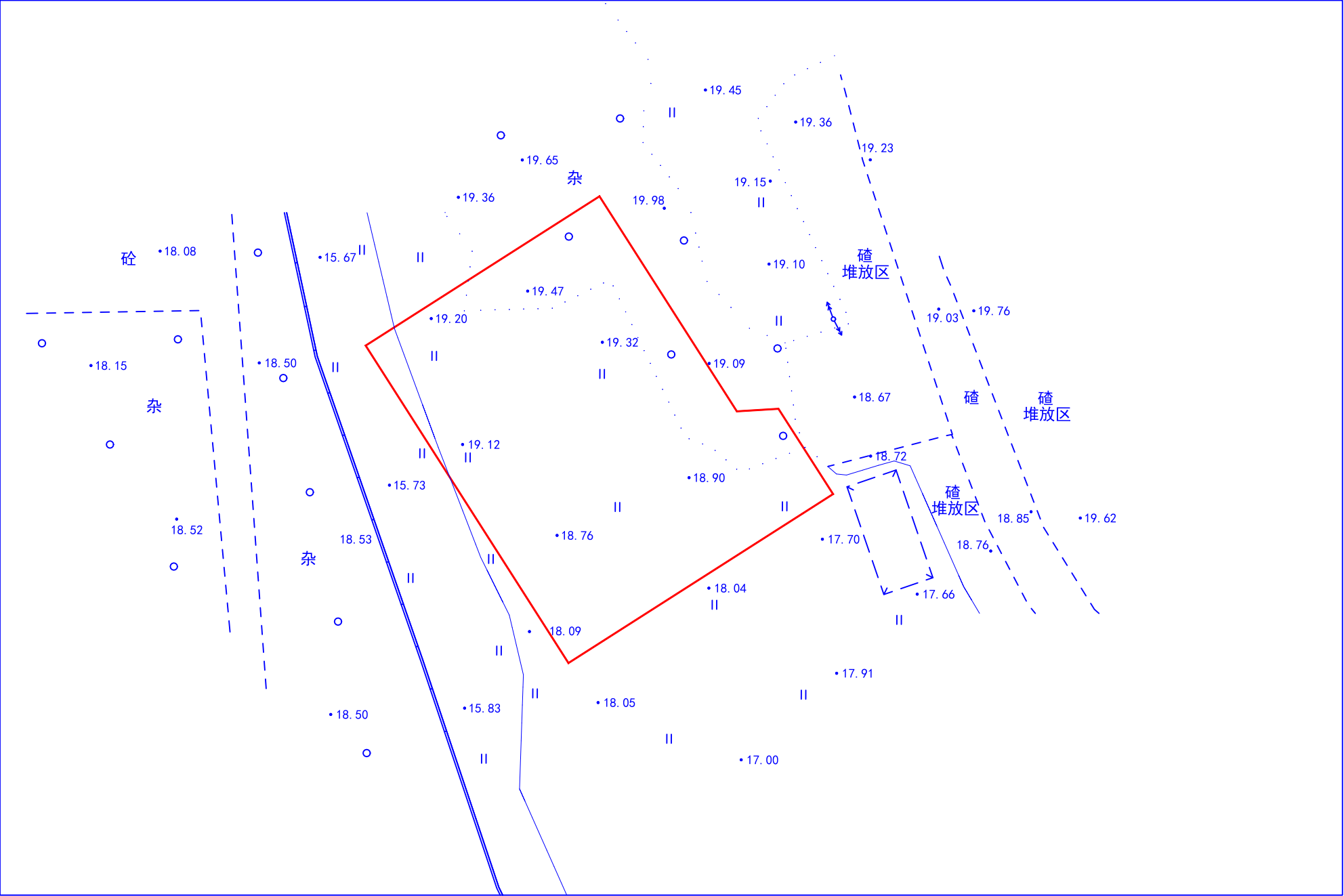
番禺区创新城净水厂进水干管（南村大道）及进水污水泵站工程-1#泵站用地地形图
