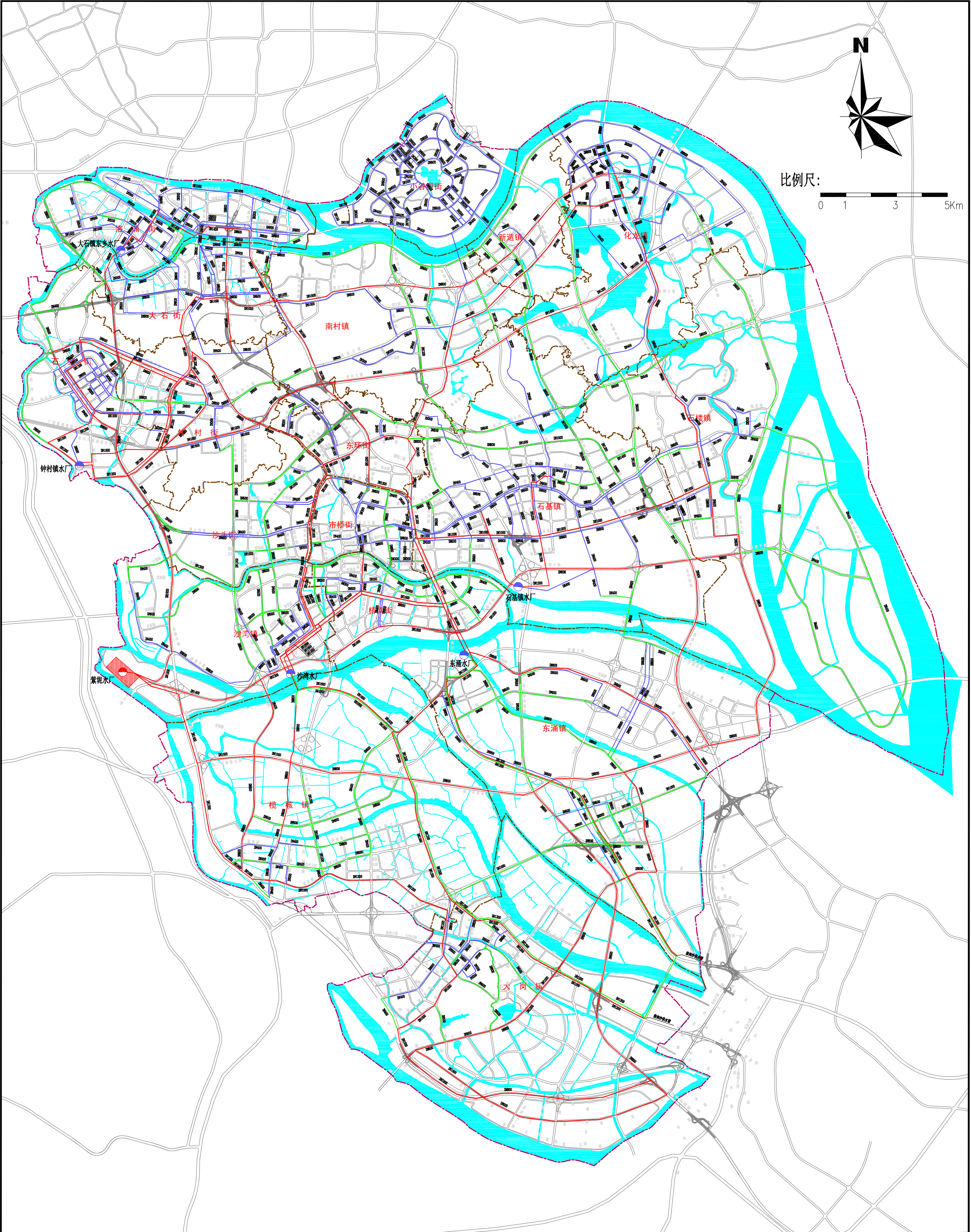
图10: 番禺区规划供水管网布置图
